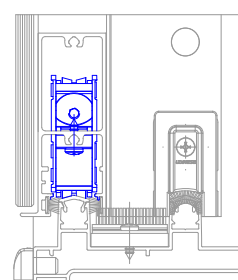
Detalhe de Aplicação Sem Escala
